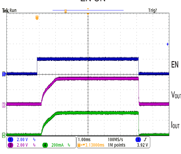
EN ON
