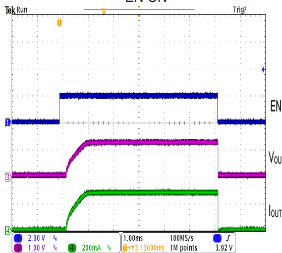
EN ON
